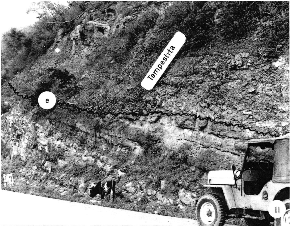
Fig. 4. Imagen del afloramiento de la capa carbonática más baja de la formación Patieccitos superior. De base a tope, se observan intercalaciones de areniscas de grano grueso, calcarenitas y calizas biogénicas, cubiertas con contacto erosional (e), por conglomerados calcáreos bioclásticos, donde abundan corales y esponjas calcáreas : D. winkleri n. sp.. El tope de la sección la forman areniscas gradadas, de grano grueso, los cuales a su vez, poseen bases erosivas, que no son evidentes en la foto. Estas secuencias heterolíticas no se repiten en la formación San Luis suprayacente.
