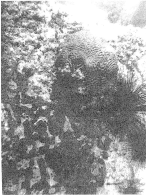
Fig. 7. Isla de Monos, costa septentrional, a 8 metros de profundidad. Fondo de substrato calcáreo, que sustenta una fauna biodiversa de corales ( Diploria strigosa ), balanidos, equinodermos ( Diadema antillarum ) y esponjas incrustantes, coloniales, que oponen poca resistencia a las corrientes fuertes, presentes en permanencia en el área. Nótese la transparencia del agua.
