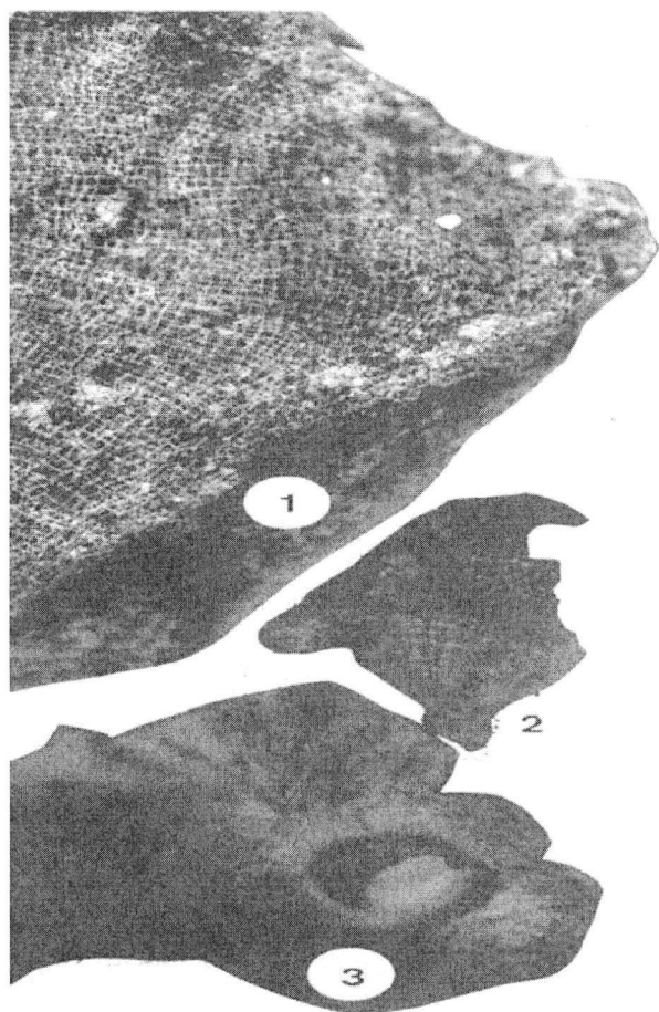
Fig. 8. Hexactinélidos o silicospongas, dragadas de la Cordillera de Aves.
